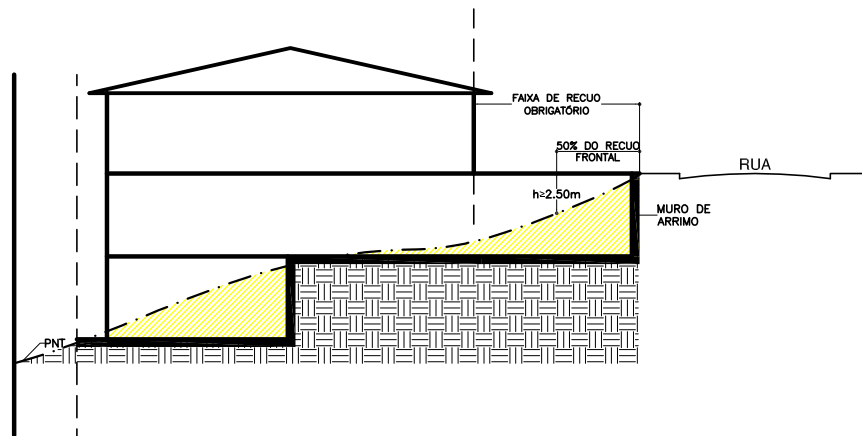
CORTE ESQUEMÁTICO AA SEM ESCALA
